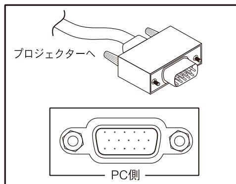
[mini D-sub 15 pin] コネクタ形状
